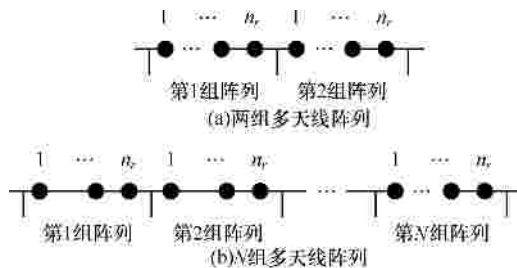
图 6 s=0 时多组多天线阵列合并方案
