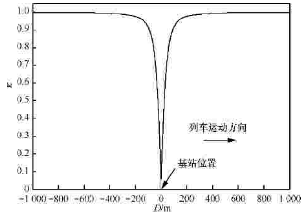
图 10 角度因子 k 的变化
