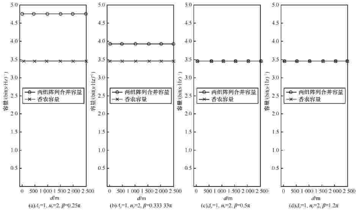
图 8 两组 D_1=1 、 n_r=2 的多天线阵列在不同权重下的容量
